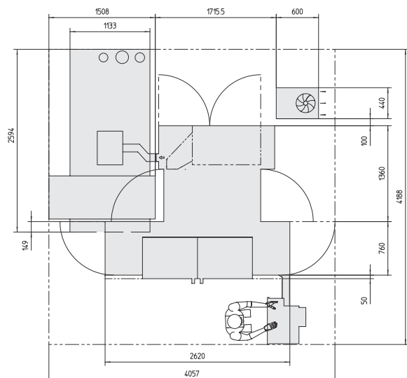
Aufstellplan 600
